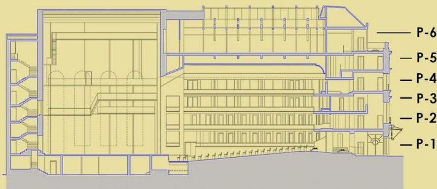
Ámbito de actuación - Sección longitudinal
